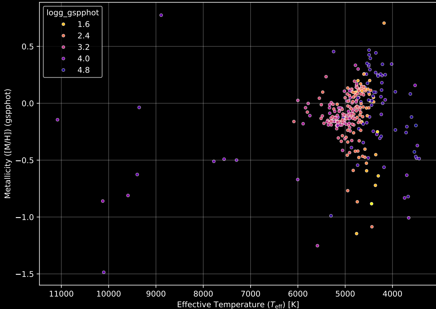
APOGEE DR17 Field: [160-24_btx] Stellar Population Parameters (n= 312)
